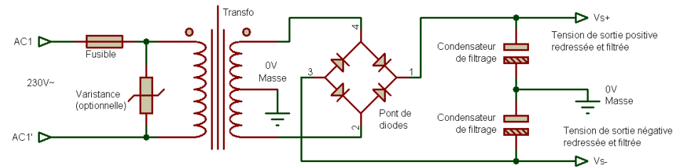
Alimentation linéaire
