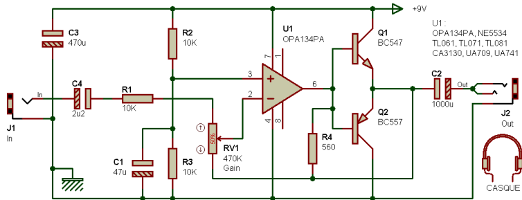
Amplificateur audio classe A
