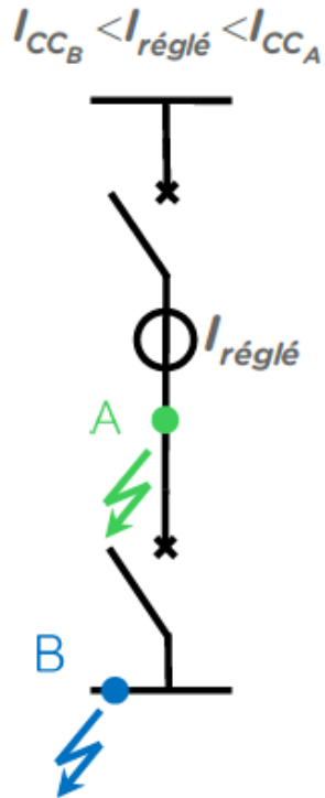
Sélectivité ampèremétrique
