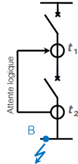
Sélectivité logique
