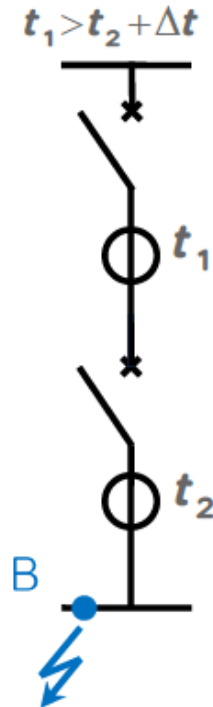
Sélectivité chronométrique
