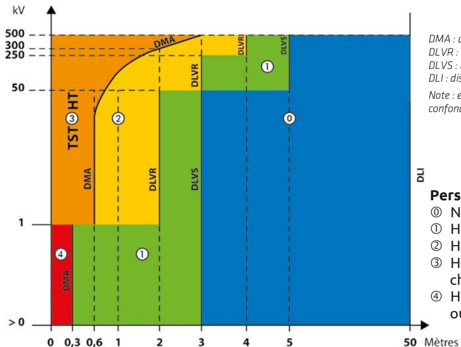
Zones de voisinage, norme NF C 18-510
