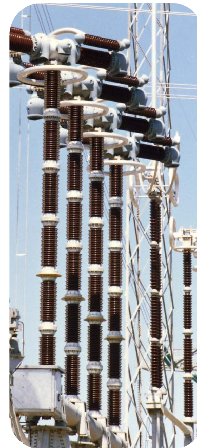
Disj. à air comprimé 2-66
