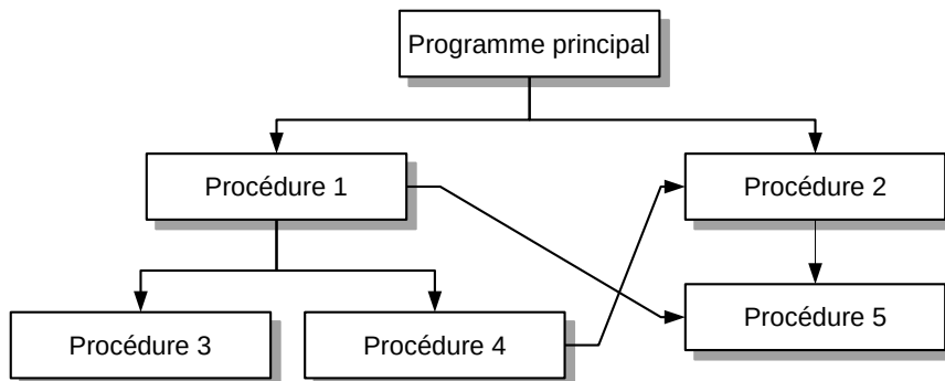
Un programme est une séquence d'appel de procédures.
